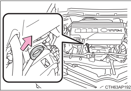
► Motor 8NR-FTS
